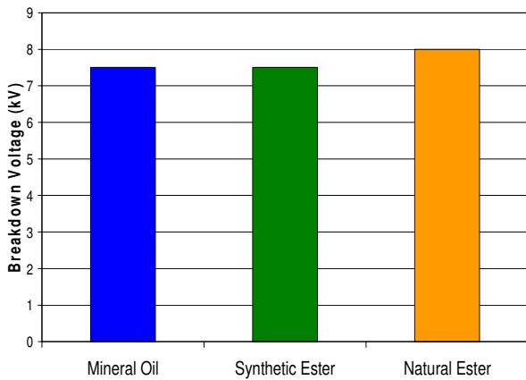
a. 90µm Kraft paper (1kV/sec)
