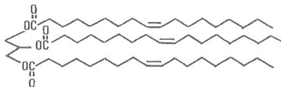
Figure 3.10 - Glyceryl tri-oleate
